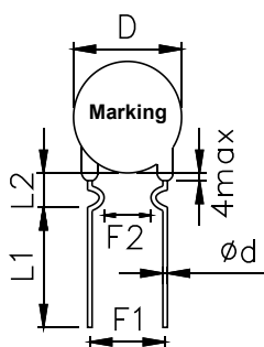
I Type (内弯脚)
